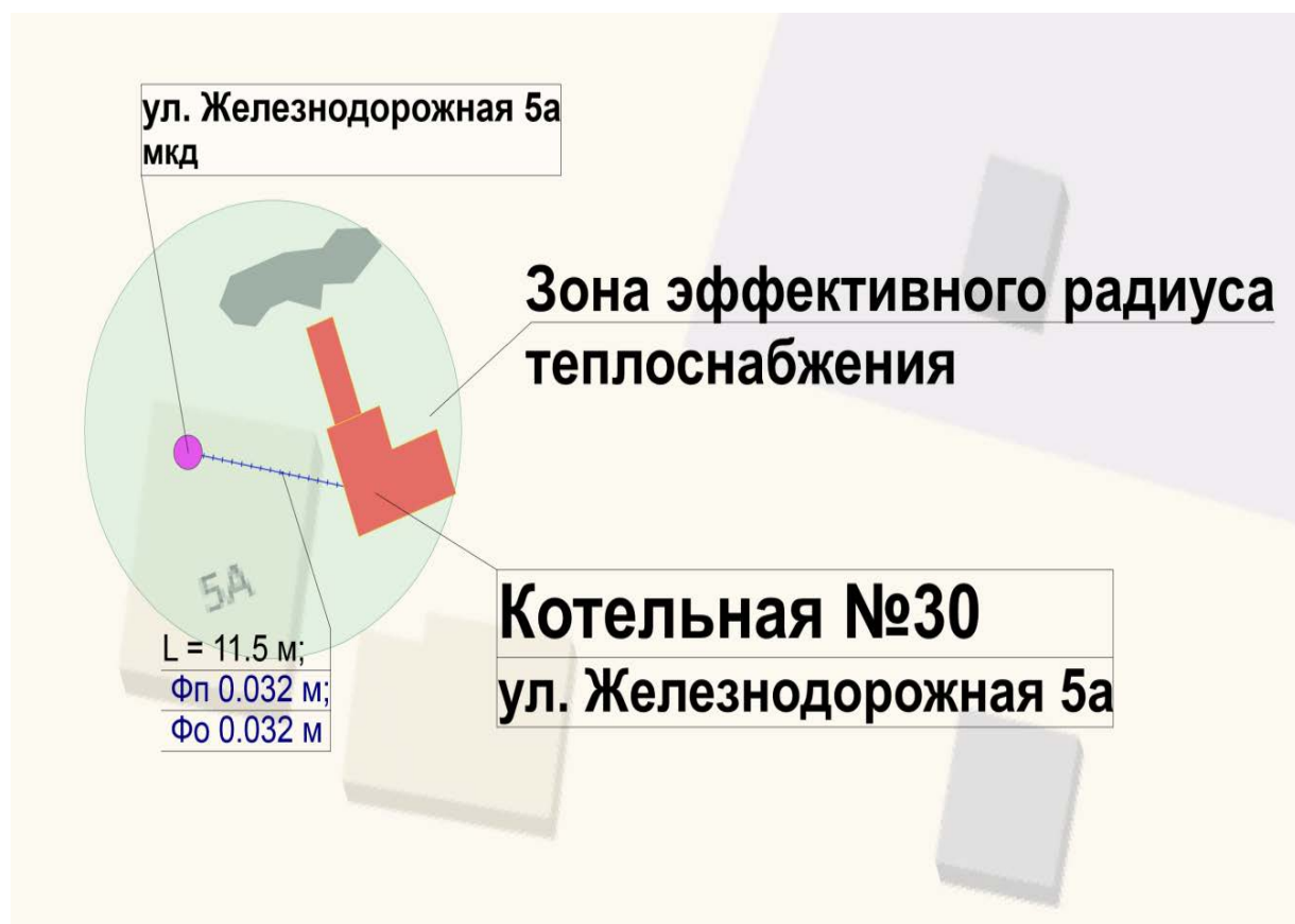
Рисунок 29. Зона эффективного радиуса теплоснабжения котельной № 30
