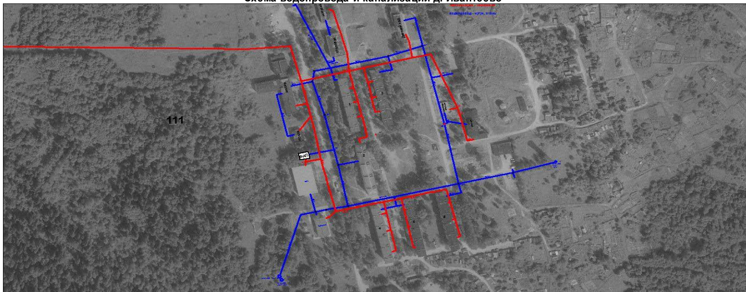
Схема водопровода и канализации д. Ивантеево
