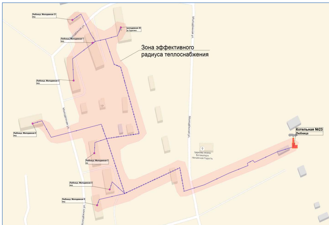
Рисунок 4. Зона эффективного радиуса теплоснабжения котельной №23
