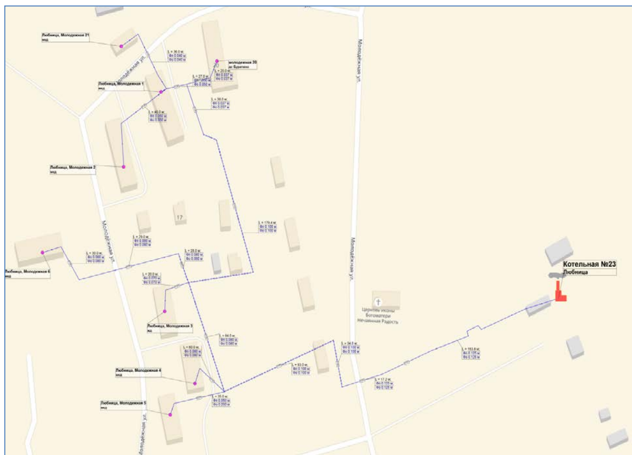
Рисунок 2. Схема тепловых сетей котельной №23 д. Любница
