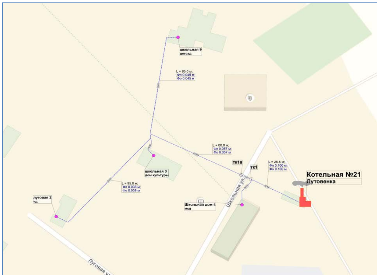
Рисунок 1. Схема тепловых сетей котельной №21, д. Лутовёнка
