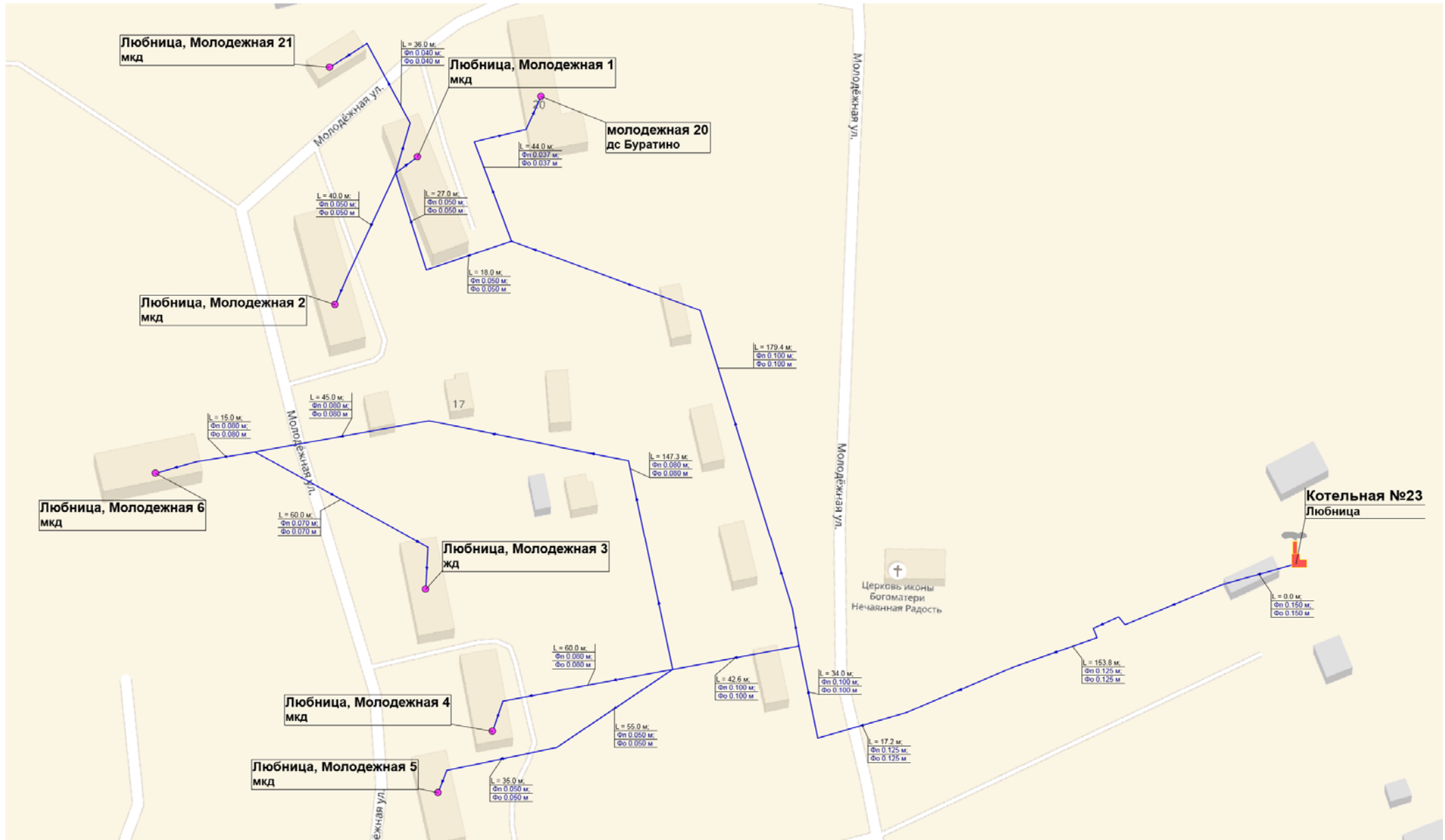
Рисунок 2. Схема тепловых сетей котельной № 23 д. Любница.
