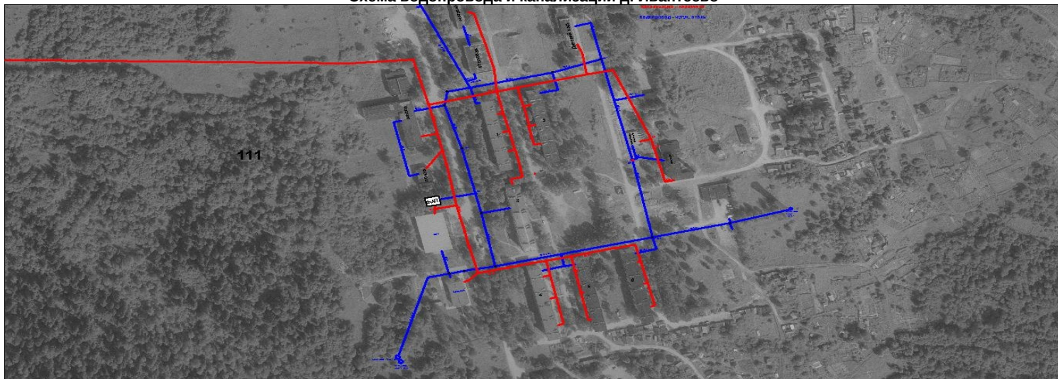
Схема водопровода и канализации д. Ивантеево
